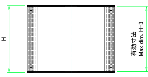
Wパネル1 / W Panel 1
