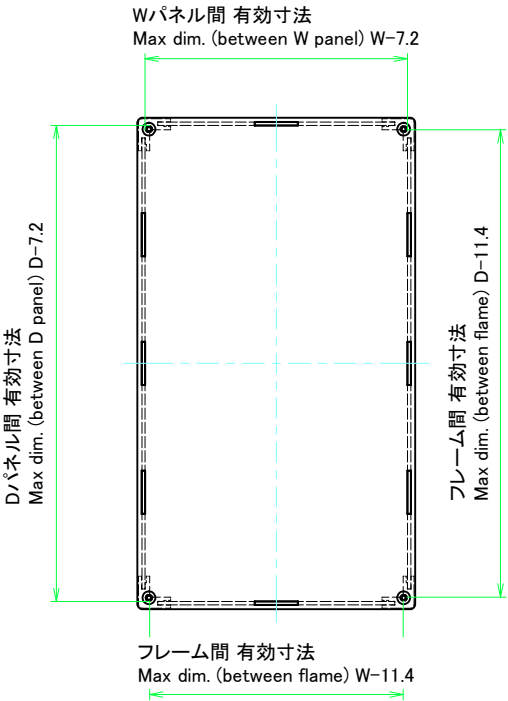
下カバー / Bottom cover
